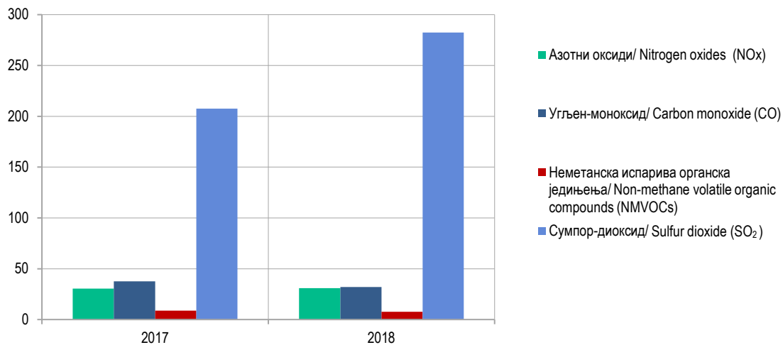
Графикон 3. Емисије индиректних гасова са ефектом стаклене баште Graph 3. Emissions of indirect greenhouse gases
