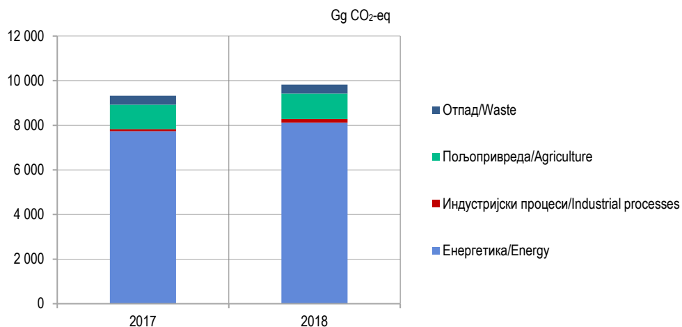
Графикон 1. Емисија директних гасова са ефектом стаклене баште (искључујући поноре), по секторима Graph 1. Direct greenhouse gas emissions (excluding sinks), by sectors
