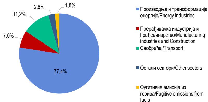
Графикон 2. Структура емисије гасова са ефектом стаклене баште из Енергетике, по подсекторима, 2018. Graph 2. Structure of the of greenhouse gas emissions from Energy, by subsectors, 2018
