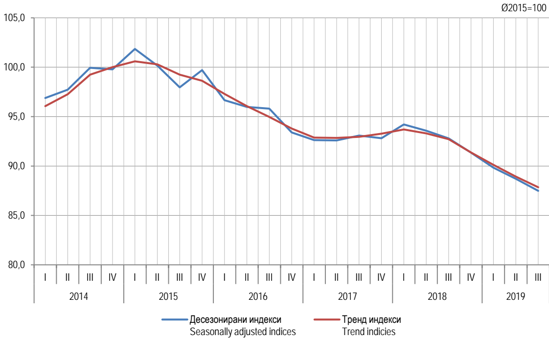
Графикон 1. Индекси производње у грађевинарству, I тромјесечје 2014 – III тромјесечје 2019. Graph 1. Indices of production in construction, 1 st quarter 2014 – 3 rd quarter 2019
