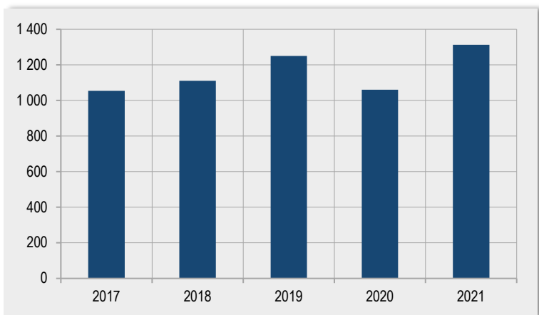
Графикон 1. Број основаних пословних субјеката
