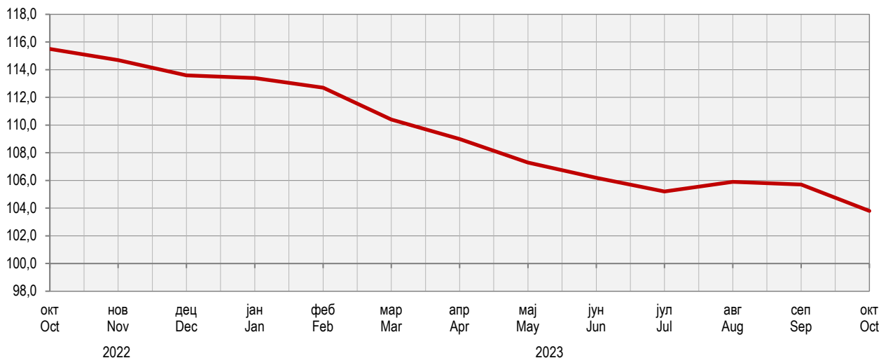
Графикон 6. Индекси потрошачких цијена, исти мјесец претходне године = 100 Graph 6. Consumer price indices, same month of the previous year = 100
