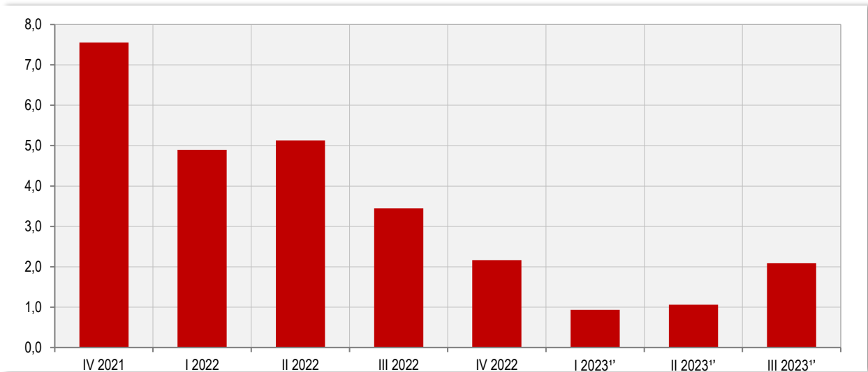
Графикон 5. Стопе реалног раста БДП-а, промјене у односу на исто тромјесечје претходне године Graph 5. Real growth rates of GDP, changes compared to the same quarter of the previous year
